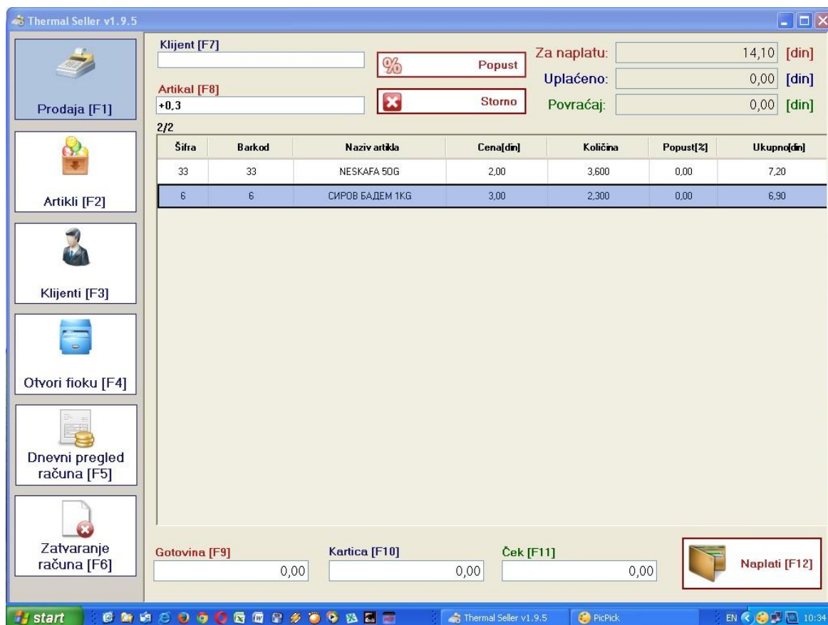
Slika 3.4 – Dodavanje količine
