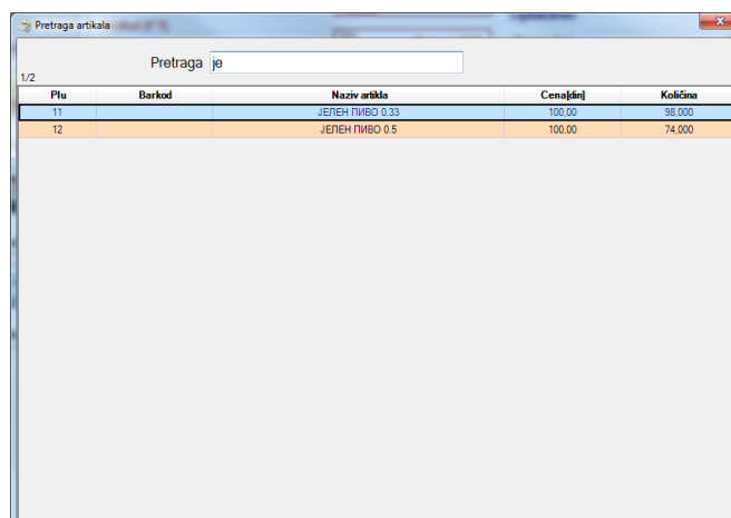
Slika 3.2 – Pretraga artikala
