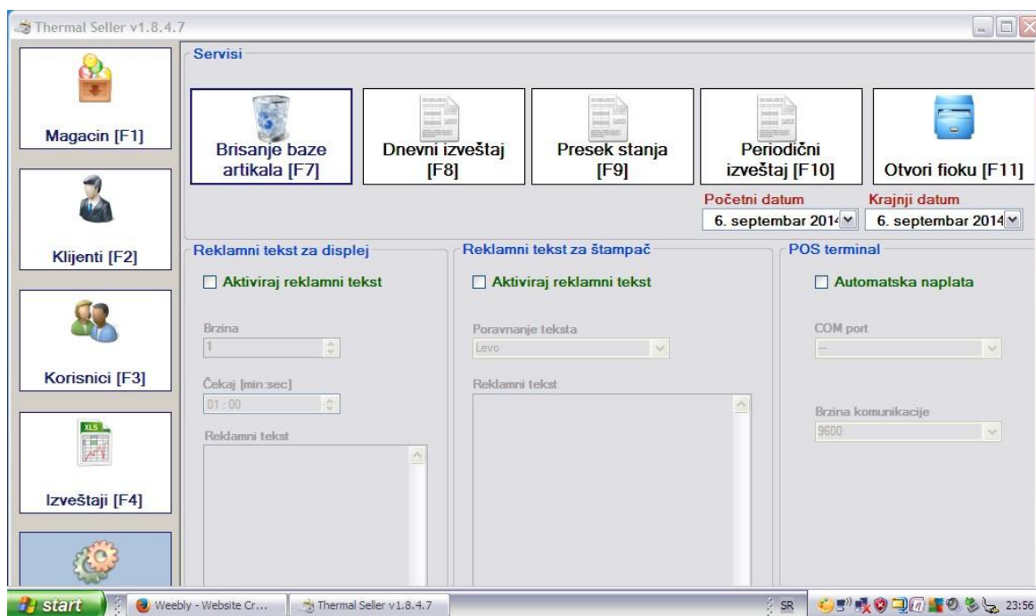
Slika 2.8 – Dodatni servisi
